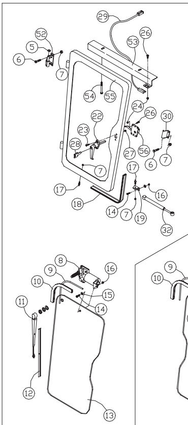
Right Hand Door Configuration
