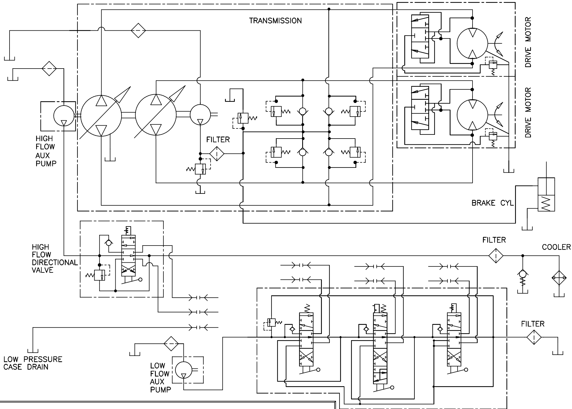
4810 HYD SCHEMATIC
